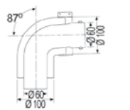
Codo 90°
