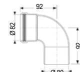
Codo 90° Ø 80
