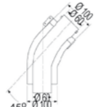
Codo 45° (2 unidades)
