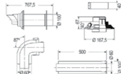
Kit salida realizada (boquilla + prolongador 0,5 m + codo 90° + terminal horizontal)
