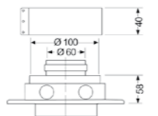
Boquilla para salida vertical o realizada con tomas de análisis
