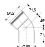
Codo 45° (2 unidades) Ø 80
