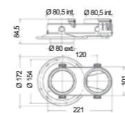
Adaptador doble flujo
