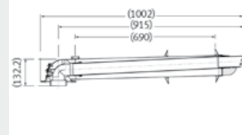
Ventosa horizontal
